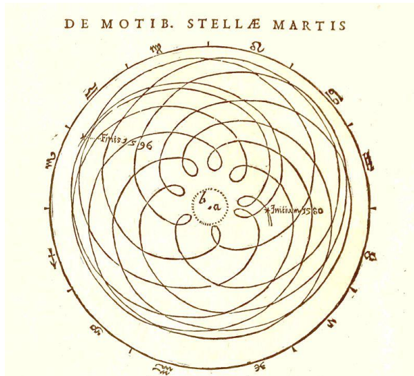
Description de Johannes Kepler des mouvements géocentriques de Mars, Astronomia nova (1609).
