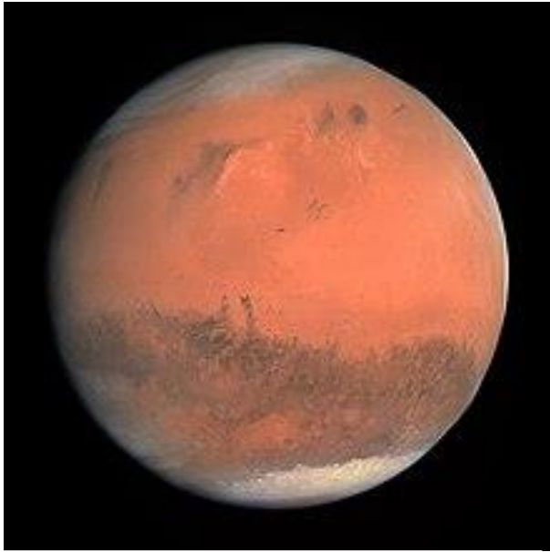
La planète Mars vue par la caméra OSIRIS de la sonde spatiale Rosetta .
